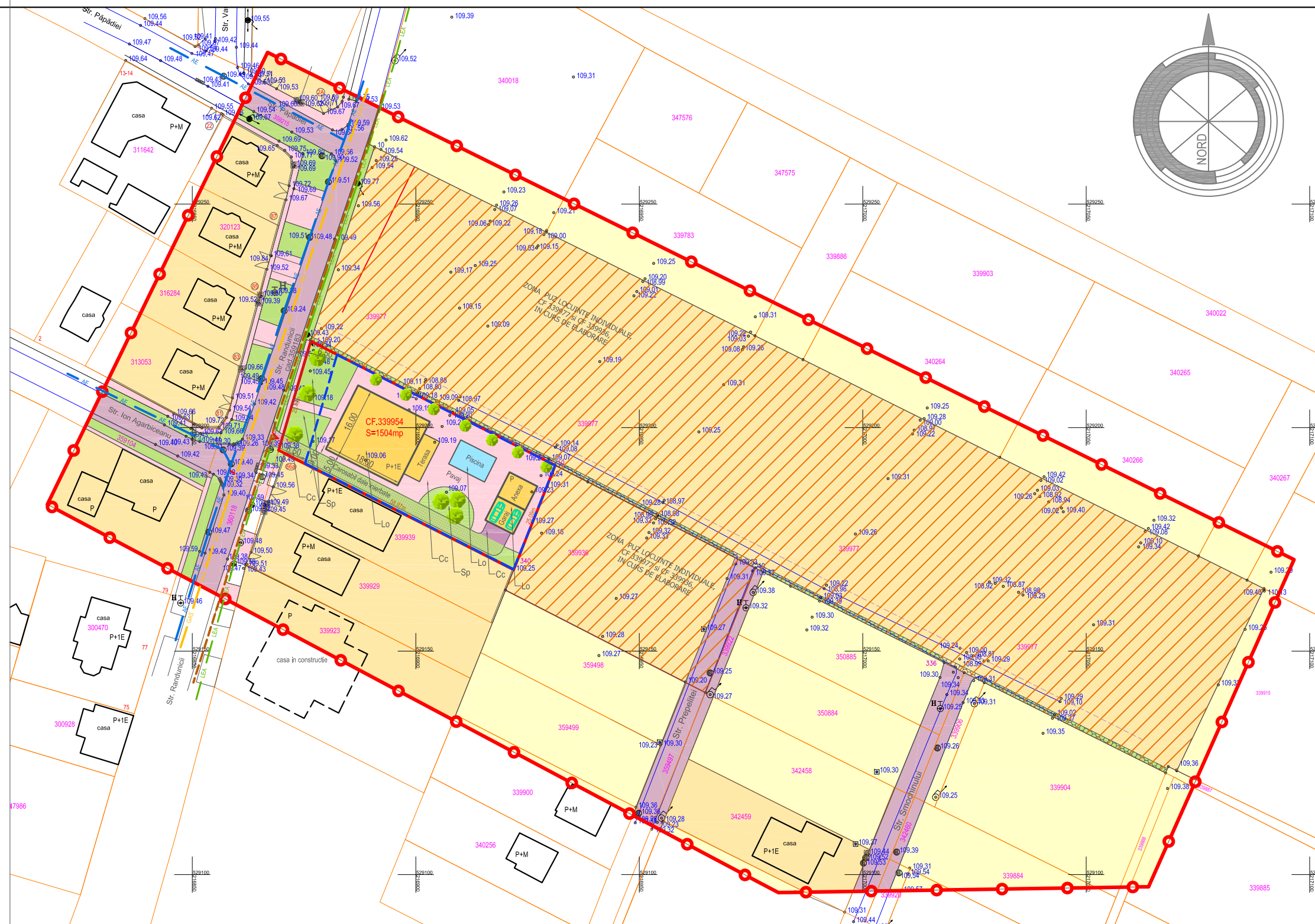
PLAN DE SITUATIE - MOBILARE DETALIU scara 1/500
