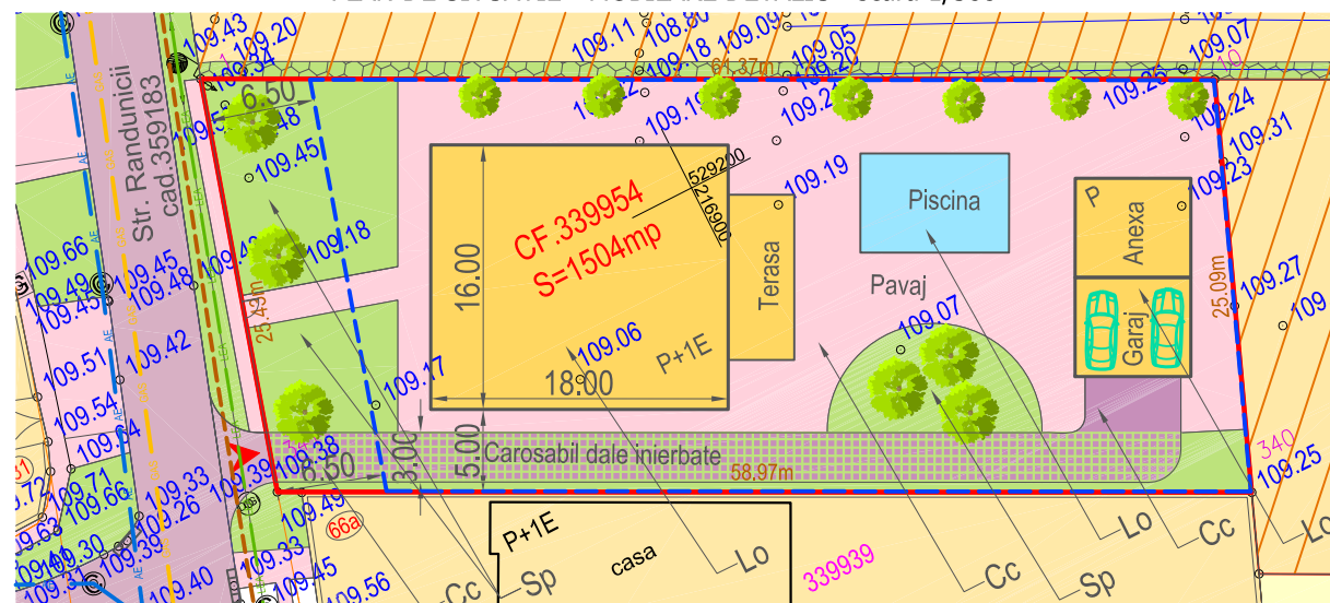
PLAN DE SITUATIE - MOBILARE DETALIU scara 1/500
