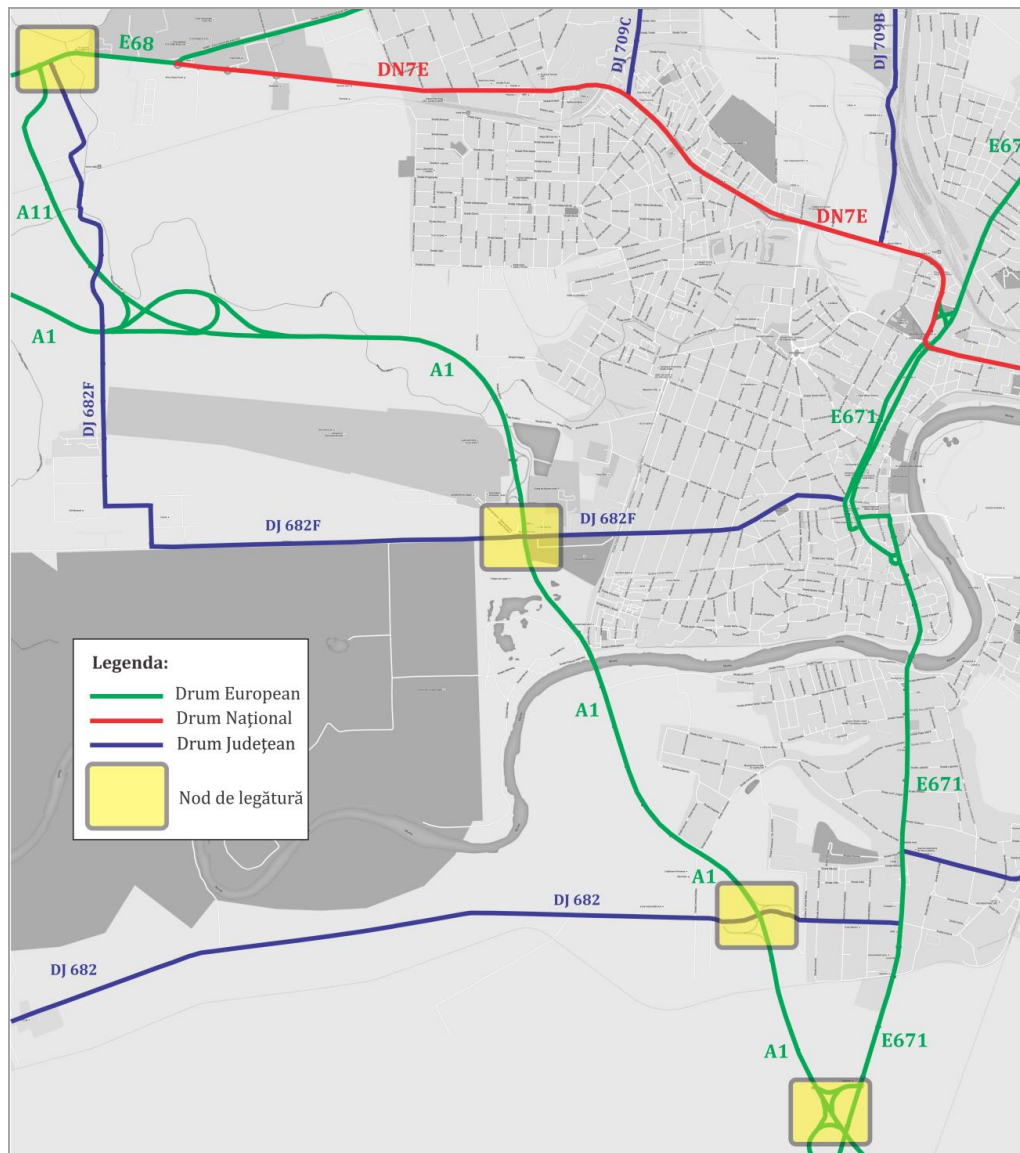
Figura 6. Nodurile de legătură ale autostrăzii A1 în zona Municipiului Arad.
